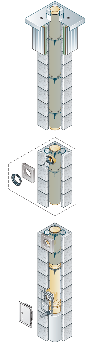
Anschluss-Variante Öl & Gas
