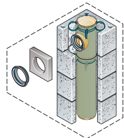
Anschluss-Variante Öl & Gas
